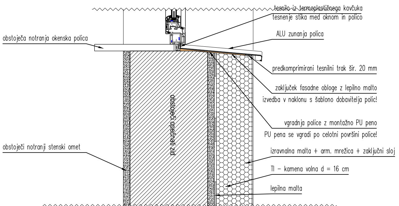
OBDELAVA OKENSKIH ODPRTIN NA OBJEKTU M 1:10 (prerez)
